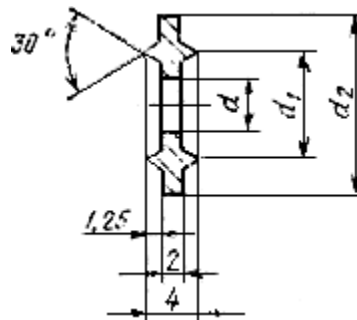
Размеры, мм
