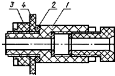
1 - гнездо сальника; 2 - шайба; 3 - гайка привертная; 4 - корпус оборудования
