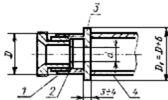
1 - гнездо; 2 - шайба; 3 - кольцо; 4 - труба
