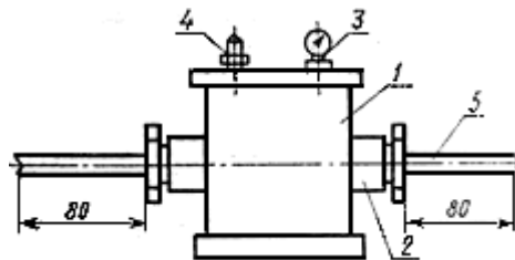
Коробка герметичная
